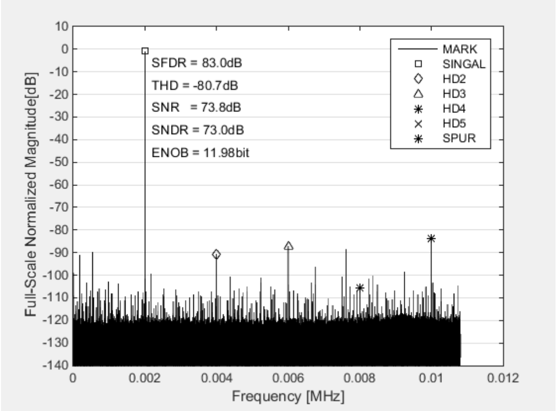
图 6-8 AC 特性@-30 摄氏度
