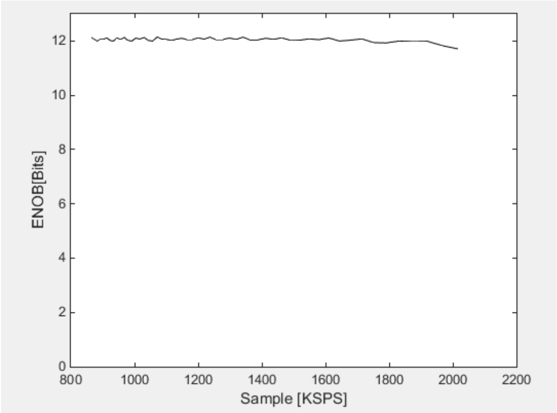
图 6-7 ENOB @转换率 (KSPS)
